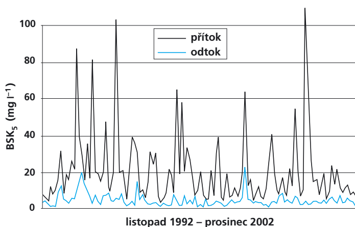
Obr. 5. Odstraňování \text{BSK}_5 na KČOV Spálené Poříčí v letech 1992–2002.
